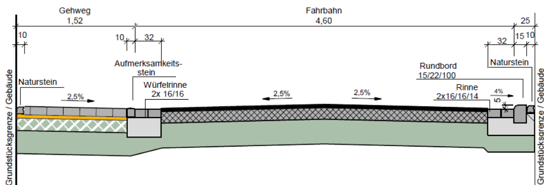
Querprofil 1 - Rathausstraße -
